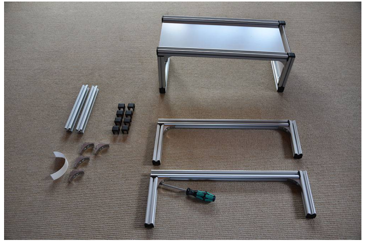
Den zweiten Seitenrahmen montieren.
